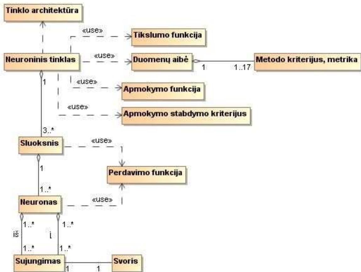
27 pav. Naudojamo daugiasluoksnio neuroninio tinklo struktūra
