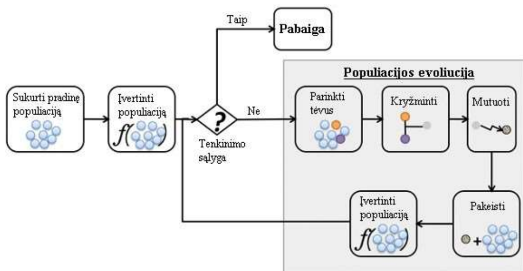
12 pav. Genetinio algoritmo struktūra [12]
