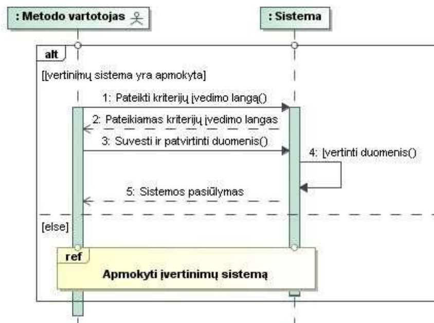
17 pav. PA „Įvertinti automatinių testų poreikį“ sekų diagrama
